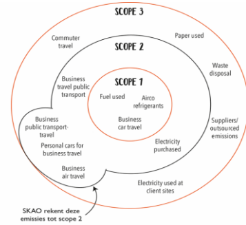
Verdeling CO 2 -uitstoot Pauw Dodewaard 2017
