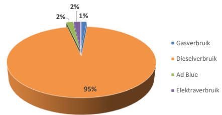
Verdeling CO 2 -uitstoot Pauw Dodewaard 2017
